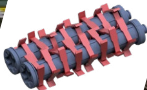
ONDES TANGENTIELLES
